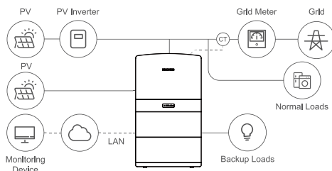
Figura 3. Sistema di accumulo ibrido accoppiato – Schema
