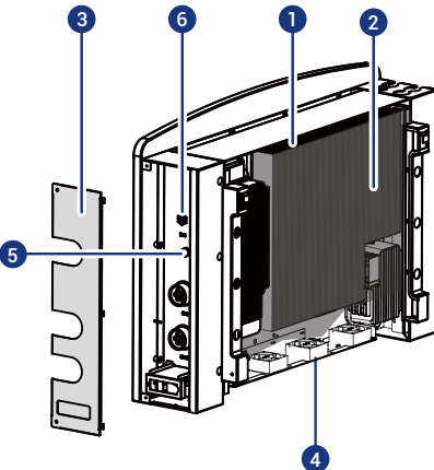
Vista esplosiva posteriore dell'inverter
