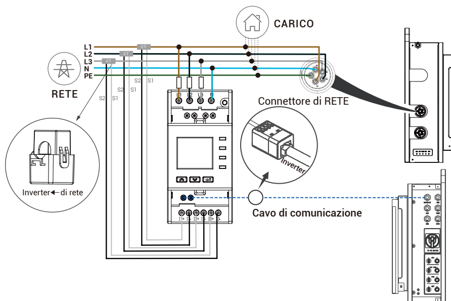
Cablaggio della connessione del contatore intelligente, esempio: ACR10RH-D16TE4 (120 A)
