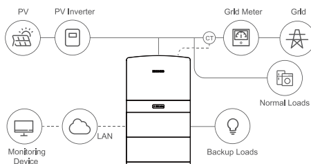
Figura 2. Sistema di accumulo accoppiato in CA – Schema
