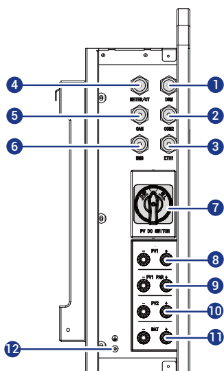
Vista sinistra dell'inverter (coperchio aperto)
