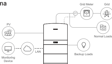
Figura 1. Sistema di accumulo accoppiato in CC – Schema
