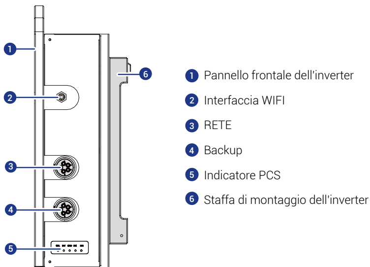
Vista lato destro dell'inverter
