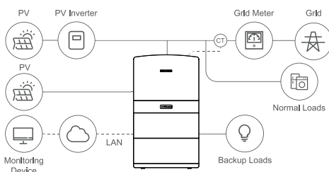
Abb. 3 Hybrid-gekoppeltes Speichersystem – Schema
