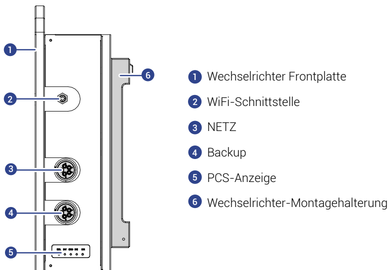
Wechselrichter-Seitenansicht rechts
