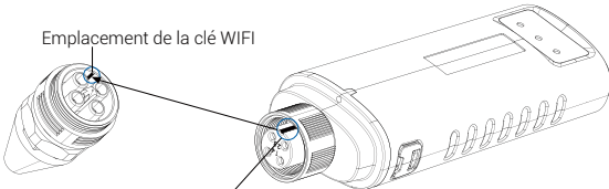
Vue arrière éclatée de l'onduleur
