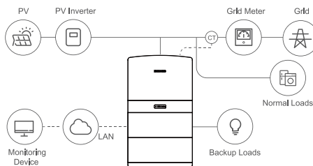
Figure 2 Système de stockage à couplage AC – Schéma
