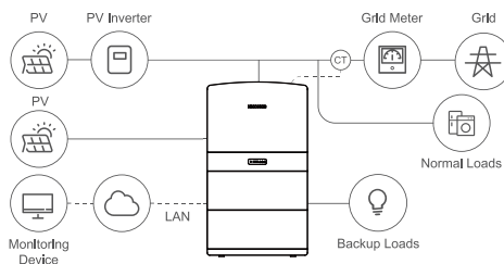
Figure 3 Système de stockage à couplage hybride – Schéma
