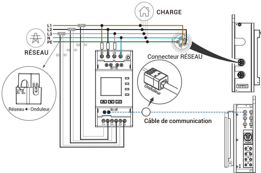
Câblage de la connexion du compteur intelligent, Exemple : ACR10RH-D16TE4 (120A)
