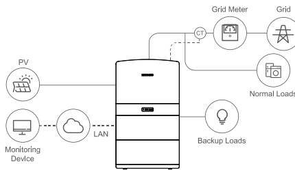
Figure 1 Système de stockage à couplage DC – Schéma
