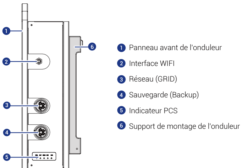
Vue latérale droite de l'onduleur
